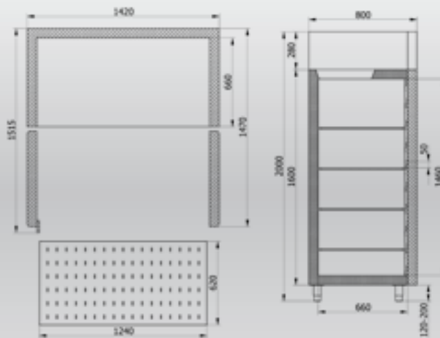
vyjímatelná kompaktní chladicí jednotka removable compact refrigerating unit
