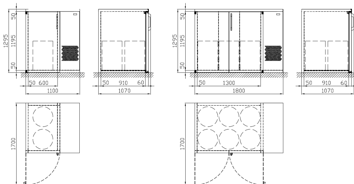
Chladicí skříně CHS-P1
